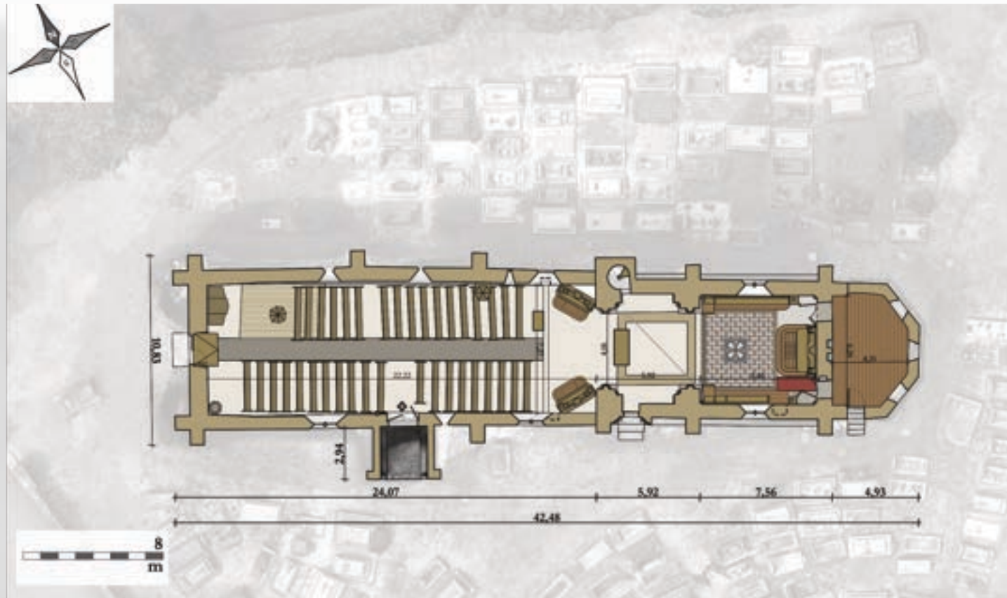
Plan de l'église
