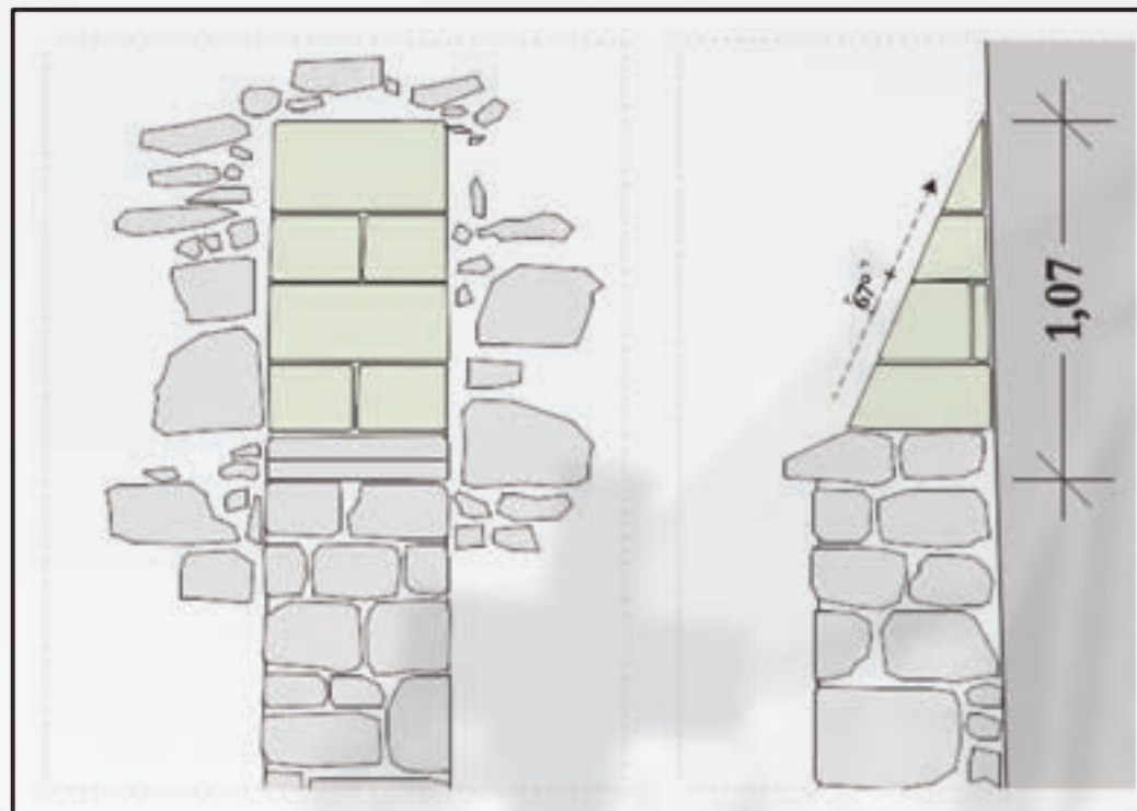
Vue de détail sur l'état projeté des glacis des contreforts de la nef.
