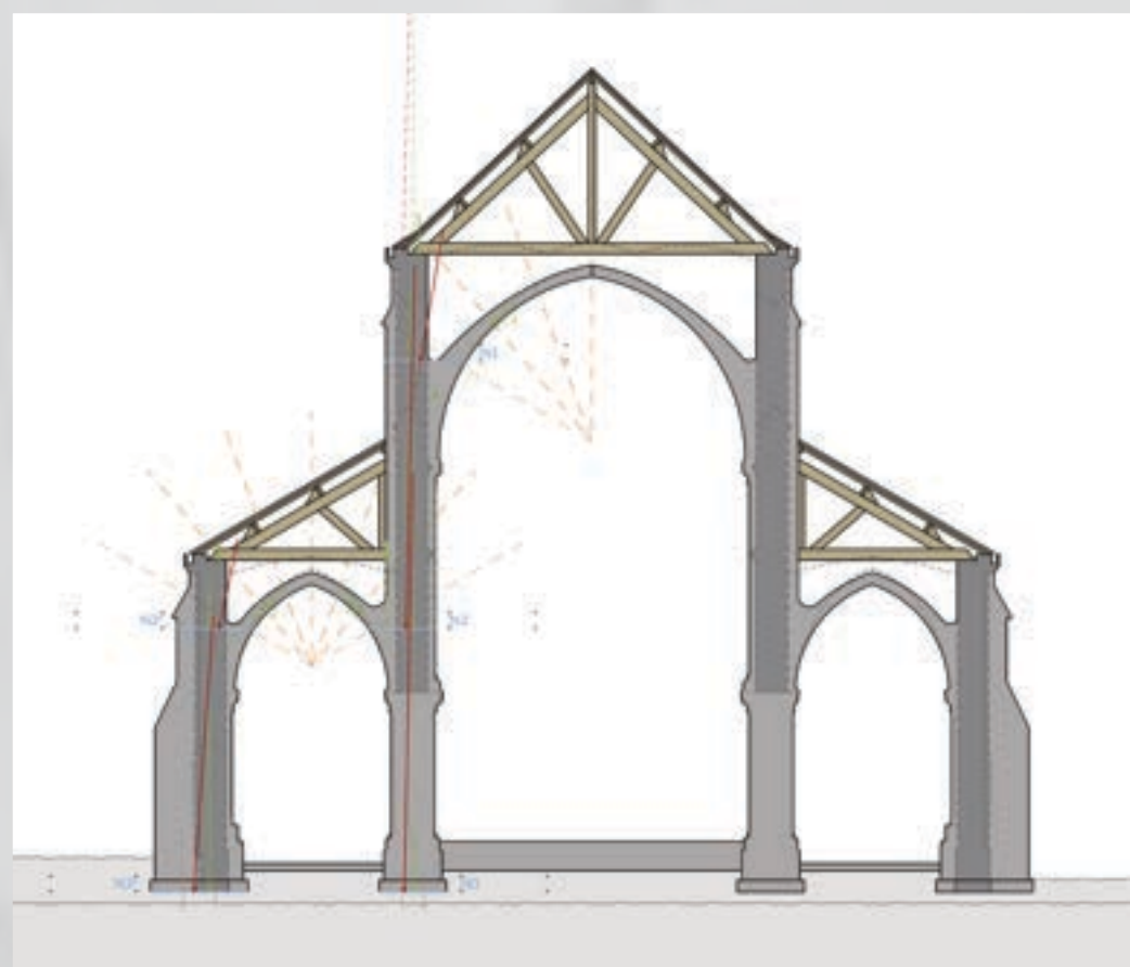
Extrait de l'épure de Mery de la nef : le but est d'étudier l'impact des descentes de charge de la structure sur les fondations.
