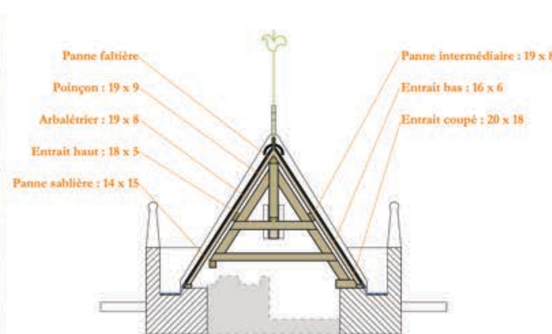
Plan de coupe projeté des couvertures du clocher.
