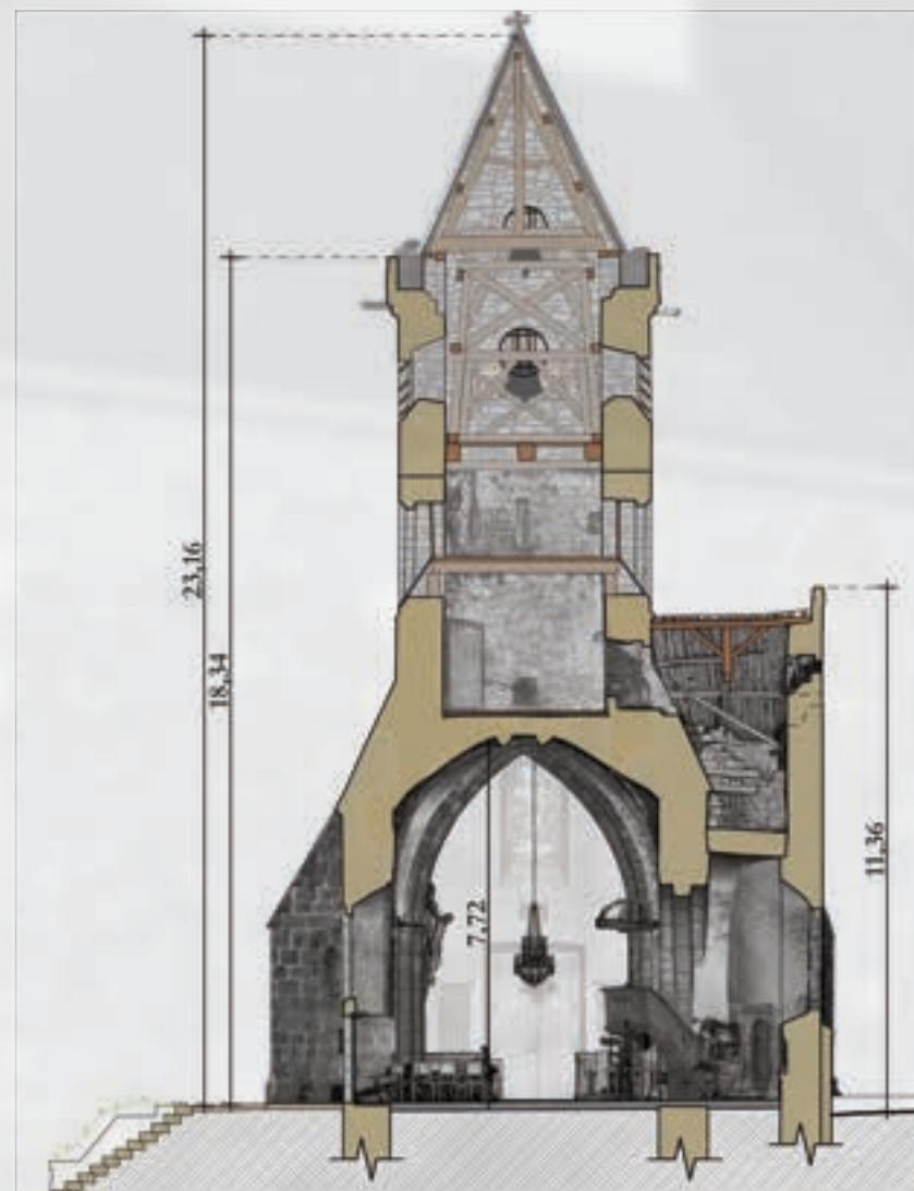
Relevé en coupe du clocher
