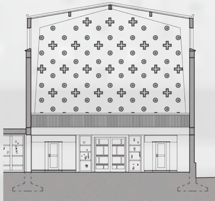
Relevé en coupe de la nef
