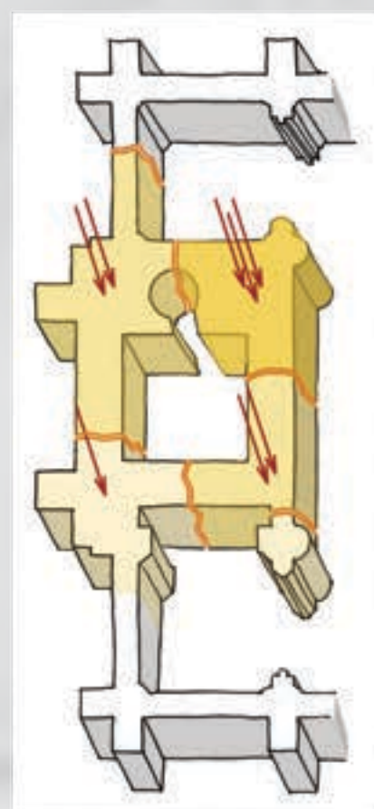
Schéma de principe montrant le tassement différentiel des fondations du clocher
