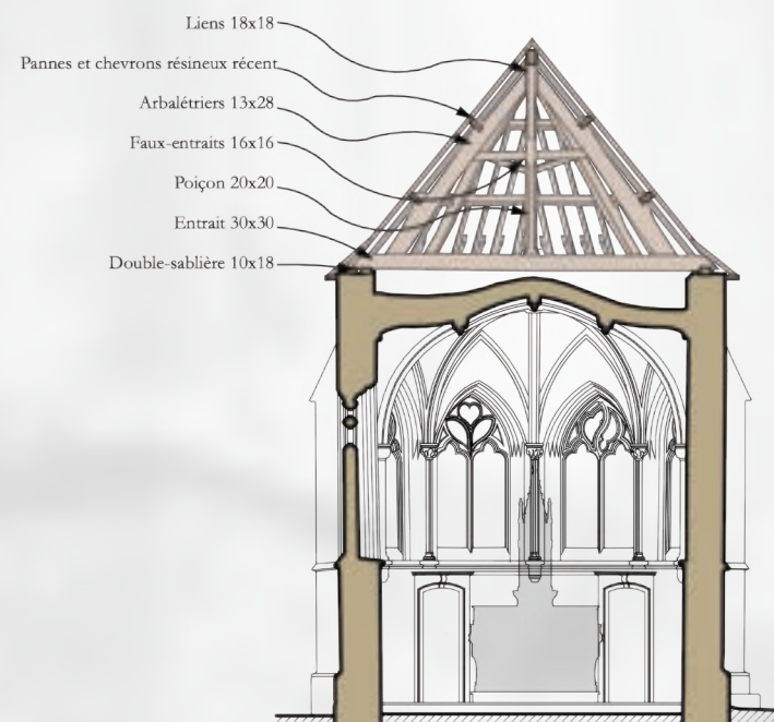
Relevé en coupe du chœur
