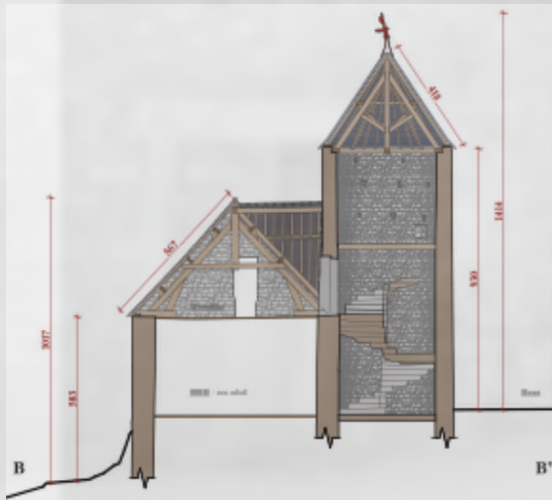
Relevé en coupe du corps de logis.
