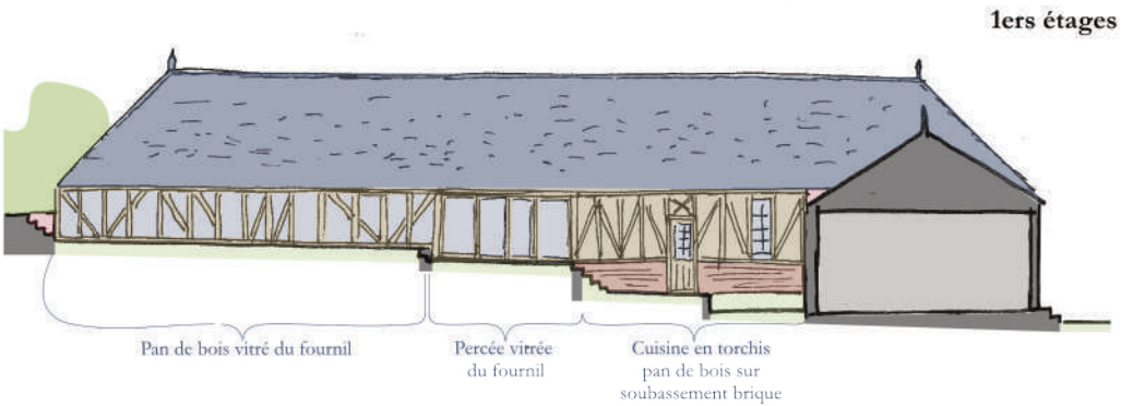
Élévation Intérieure OUEST
