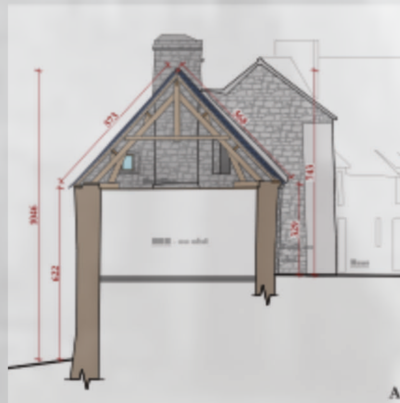
Relevé en coupe du corps de logis.
