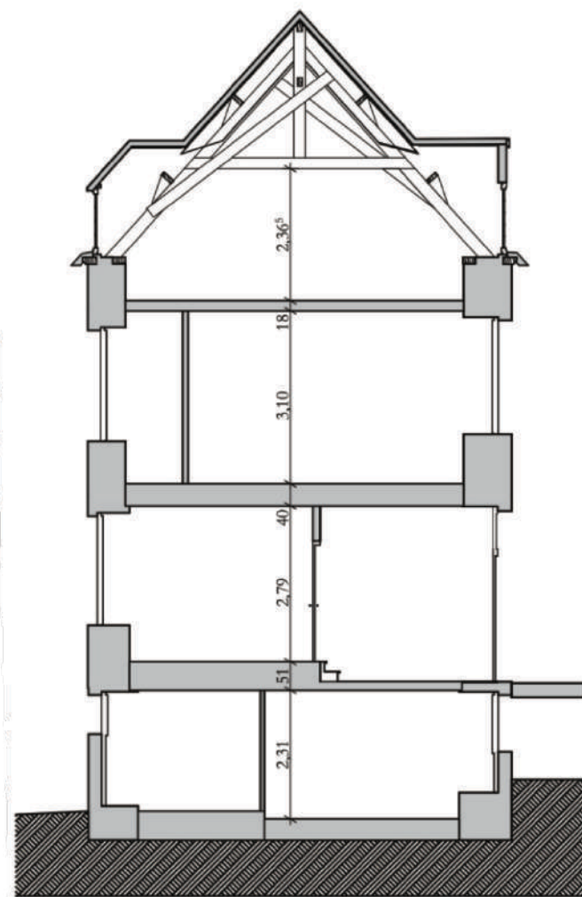
Coupe C2
